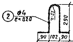
Монтажная петля
