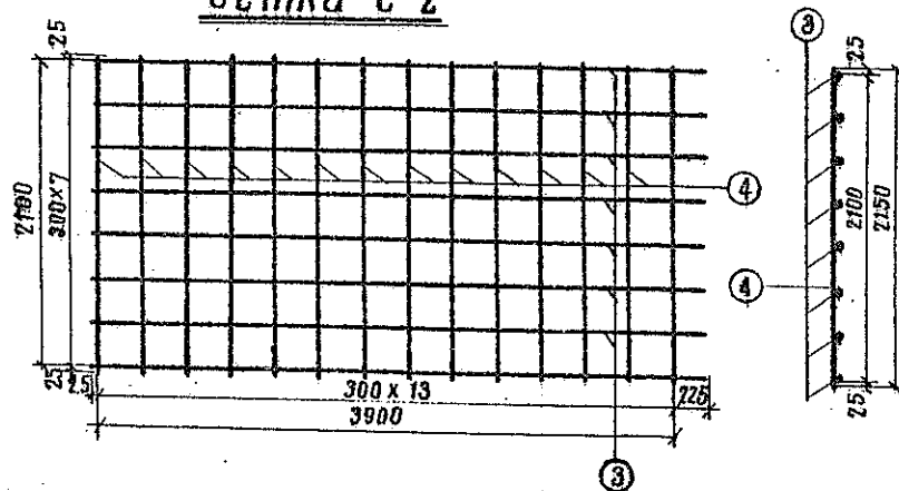
Сетка С-2
