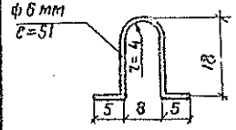
Монтажная петля
