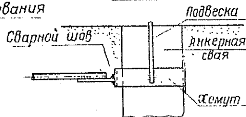
Вид по I-I
