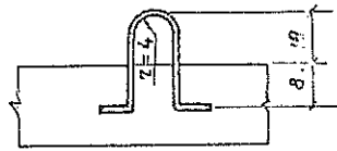
Крепление монтажной петли
